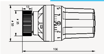
concept Thermostatkopf mit Klemmanschluss für Danfoss-Ventilunterteile der Baureihe RA Farbe: weiß Art.-Nr.: C2907312090 Farbe: chrom Art.-Nr.: C2907312002
