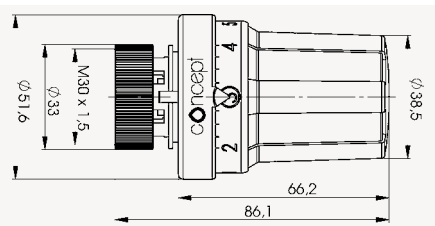
concept Thermostatkopf mit Schraubanschluss M 30 x 1,5 Farbe: weiß Art.-Nr.: C2907302190 Farbe: chrom Art.-Nr.: C2907302002
