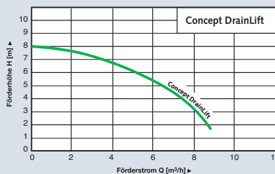
Hydraulische Daten Concept DrainLift Förderstrom: max. 8,7 m³/h; Förderhöhe: max. 8 m; Druckzulaufhöhe: 300 mm
