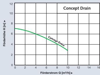
Hydraulische Daten Concept Drain Förderstrom: max. 10 m³/h Förderhöhe: 7 m
